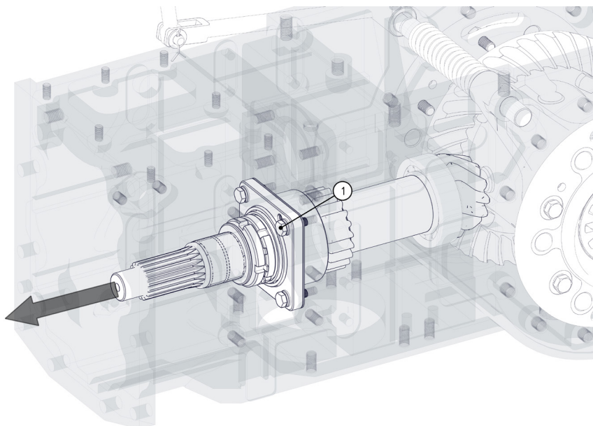
Рис. 31 Регулировка подшипников вала главной пары дифференциала
