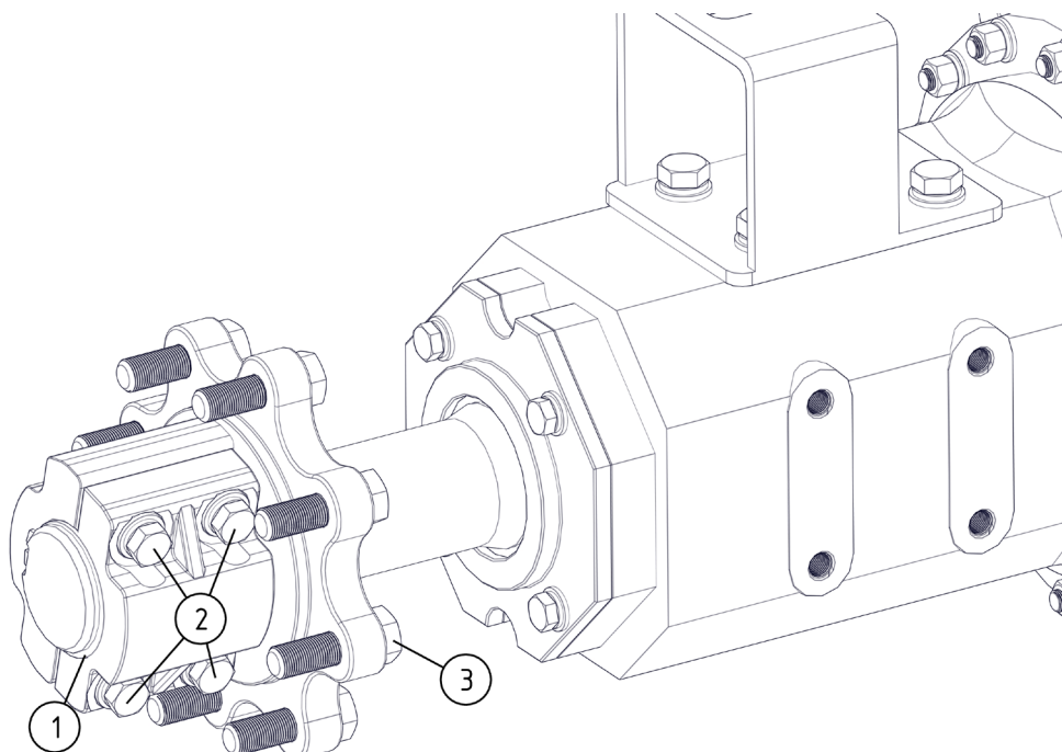
Рис. 63 Регулировка колеи задних колес
