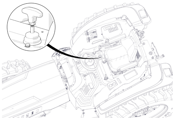
Рис. 12 Расположение рычага ходоуменьшителя
