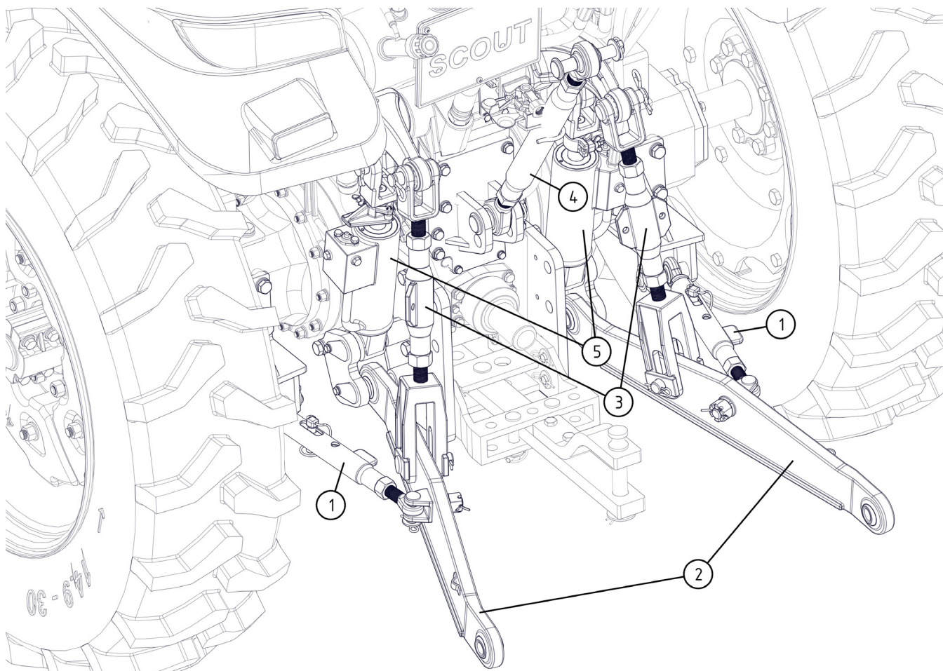
Рис. 74 Регулировка подъемного трехточечного механизма
