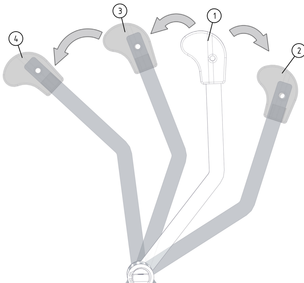
Рис. 73 Положения рычага трехточечного механизма
