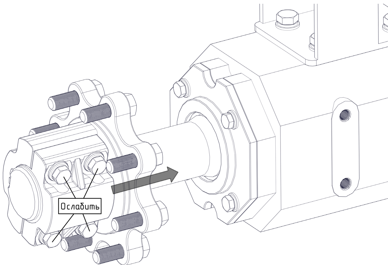
Рис. 61 Регулировка колеи задних колес
