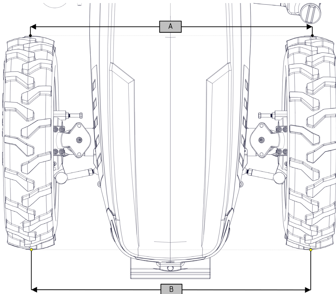
Рис. 66 Регулировка схождения передних колес трактора
