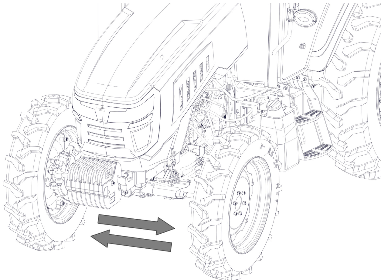
Рис. 60 Регулировка колеи передних колес перестановкой
