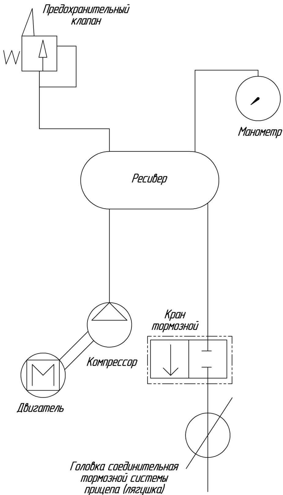
Рис. 59 Принципиальная пневматическая схема
