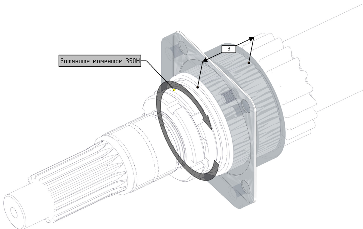
Рис. 33 Регулировка подшипников вала главной пары дифференциала
