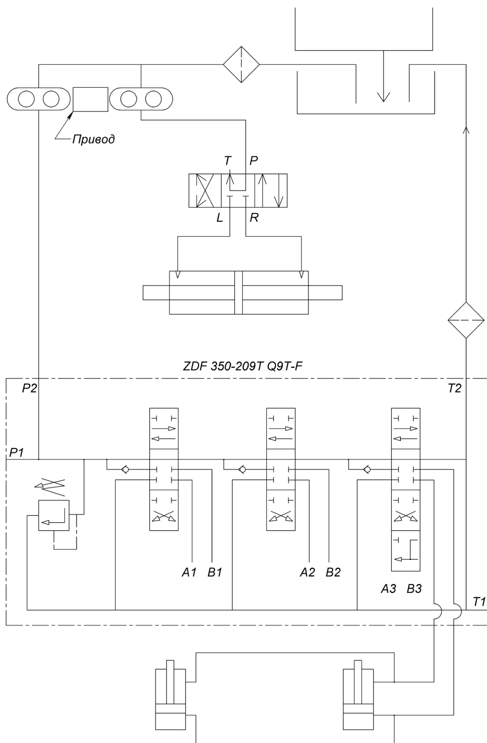
Рис. 58 Принципиальная гидравлическая схема
