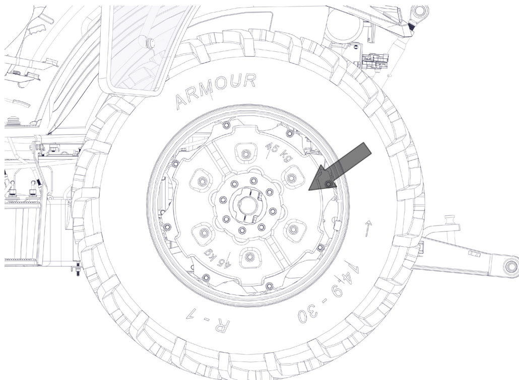
Рис. 69 Расположение задних утяжелителей
