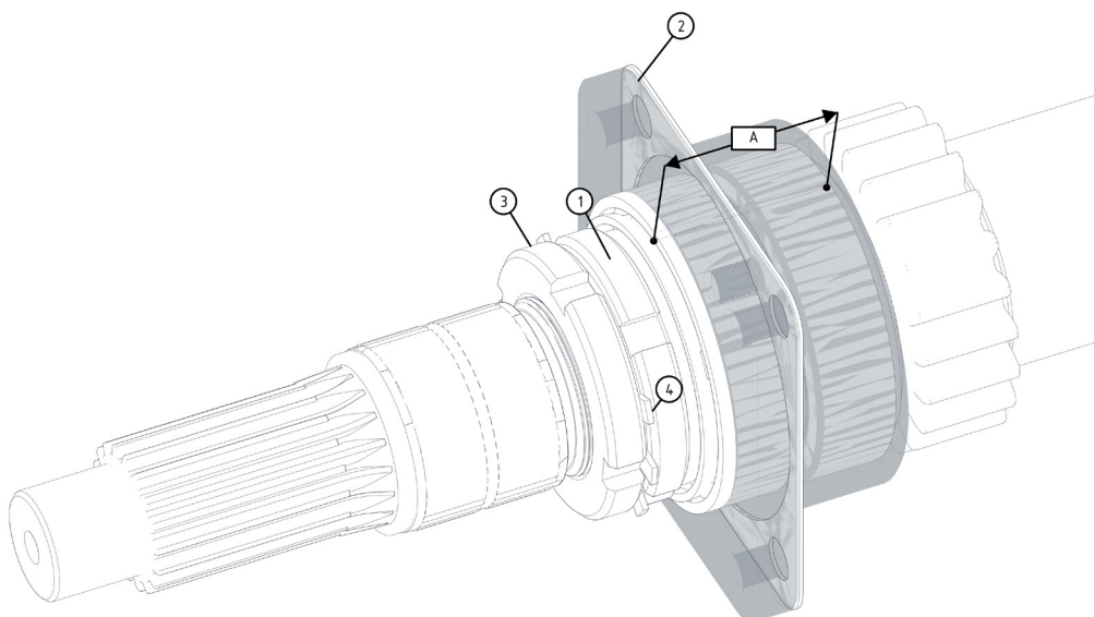
Рис. 32 Регулировка подшипников вала главной пары дифференциала
