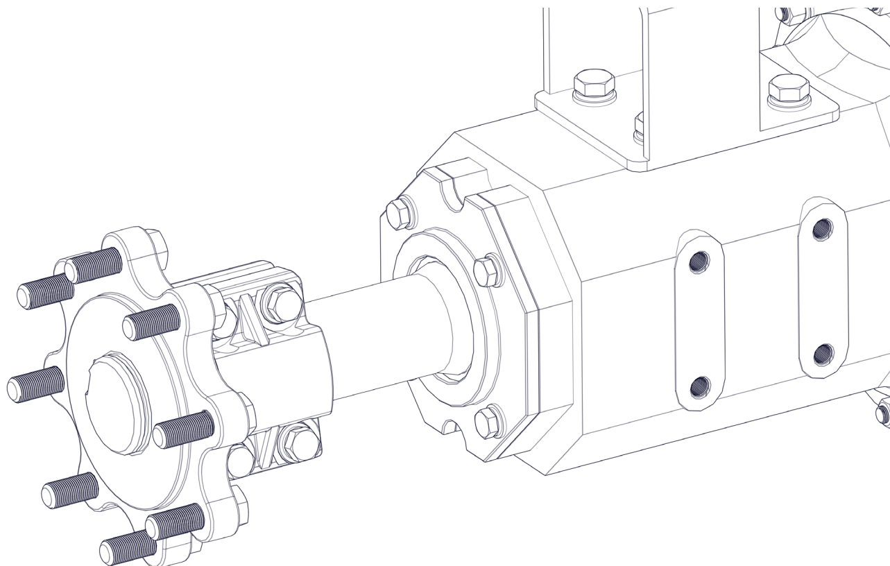
Рис. 64 Регулировка колеи задних колес
