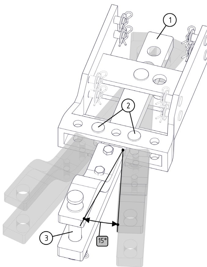
Рис. 76 Прицепное маятниковое устройство
