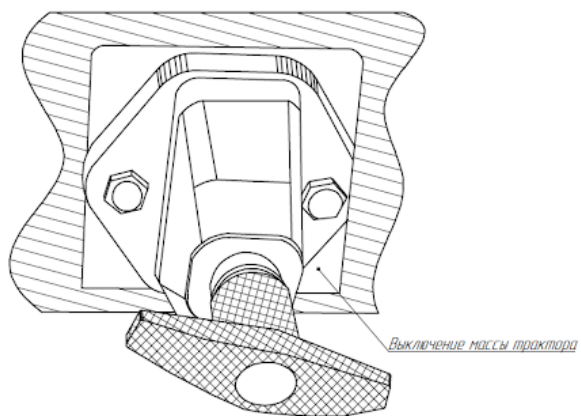
Рис. 24 Ручка включения массы трактора
