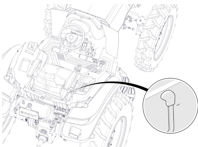
Рис. 19 Расположение рычага трехточечного механизма
